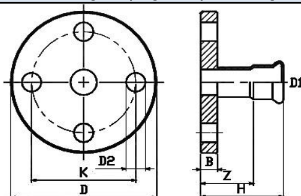
Pers overgangsfleks PN 16 pers x flens Press flange coupling PN 16 press x flange
